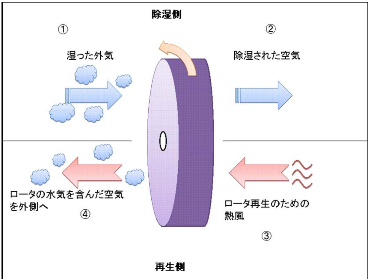
【デシカントロータの概念図】
