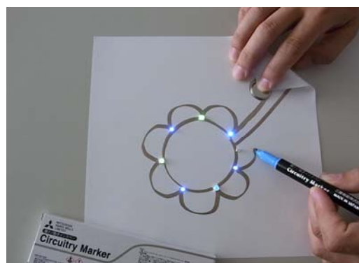
手描き電子回路でのLED発光の様子
